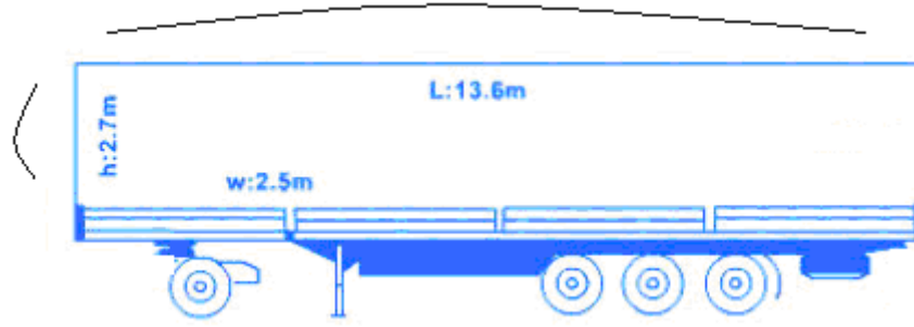
MAXİMA TİPİ SEMİ-TREYLER
