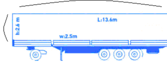
OPTİMA TİPİ SEMİ-TREYLER
